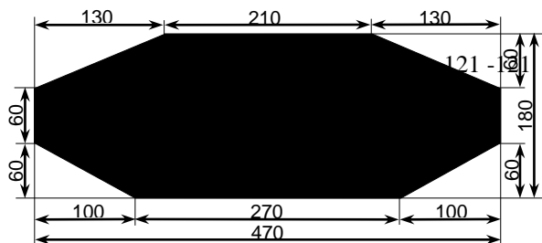
Мал. 28 БТР (мішень № 13а)
